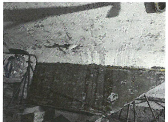
Renblästrad köl, all färg borttagen
